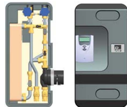
Production d'eau chaude instantanée par échangeur à plaques intégré, régulation pré-cablée et pré-réglée
