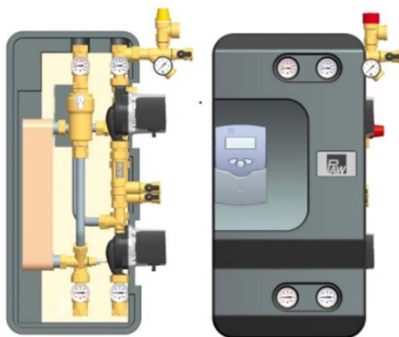
Groupe de transfert solaire complet avec échangeur à plaques, régulation pré-cablée et pré-réglée
